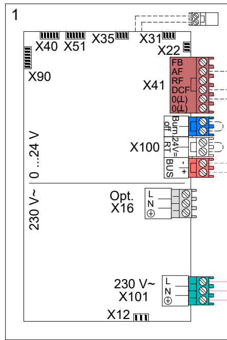
ecoTEC plus
