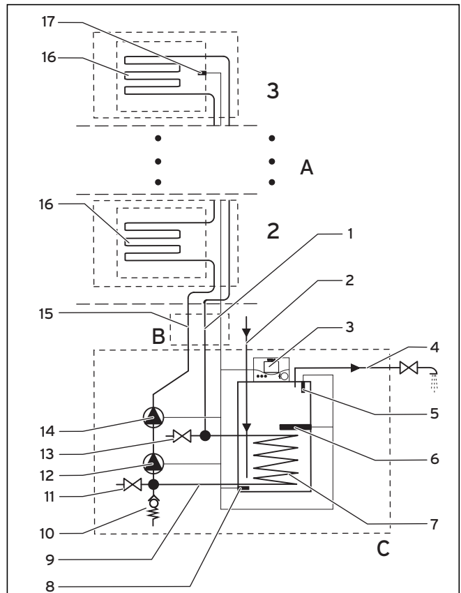
2.3 ábra VEH SN 350/3 iP bojlerrel rendelkező auroSTEP plus rendszer fő komponensei (elvi vázlat csatlakozótartozékok nélkül)
