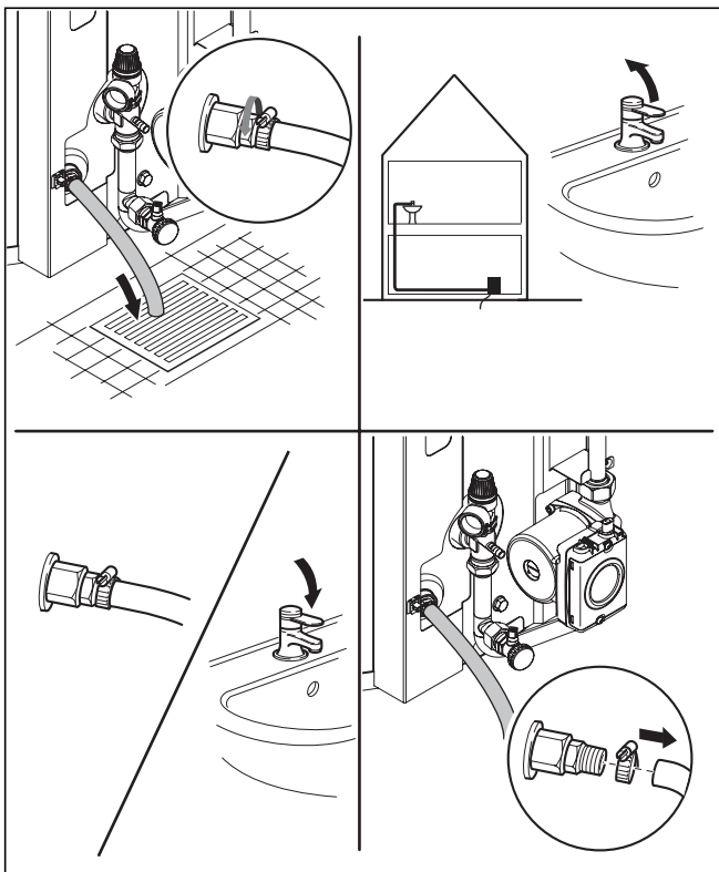
4.8 ábra A bojler kiürítése
