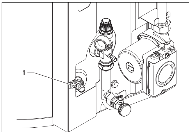
4.2 ábra A használati melegvízbojler ürítőszelepe
