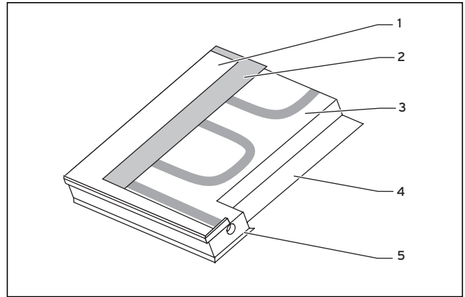
2.6 ábra A Vaillant auroTHERM classic VFK 135 D síkkollektor metszete
