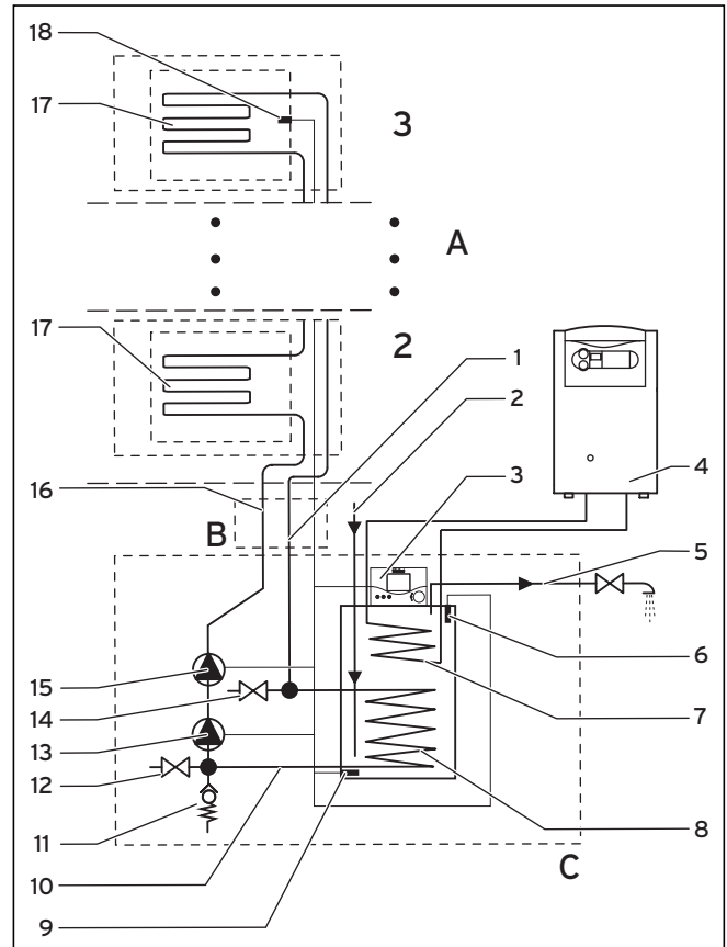
2.3 ábra VIH SN 350/3 iP tárolóval rendelkező auroSTEP plus rendszer fő komponensei (elvi vázlat csatlakozótartozékok nélkül)
