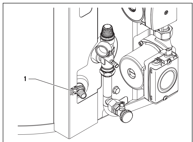
4.2 ábra A használati melegvíztároló ürítőszelepe
