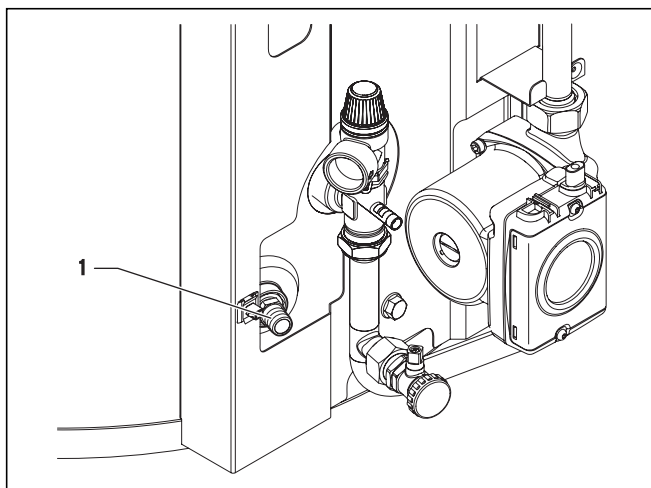
4.2 ábra A használati melegvítároló üritőszelepe
