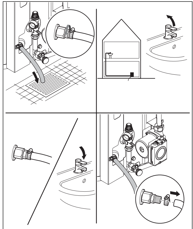
4.8 ábra A tároló ürítése
