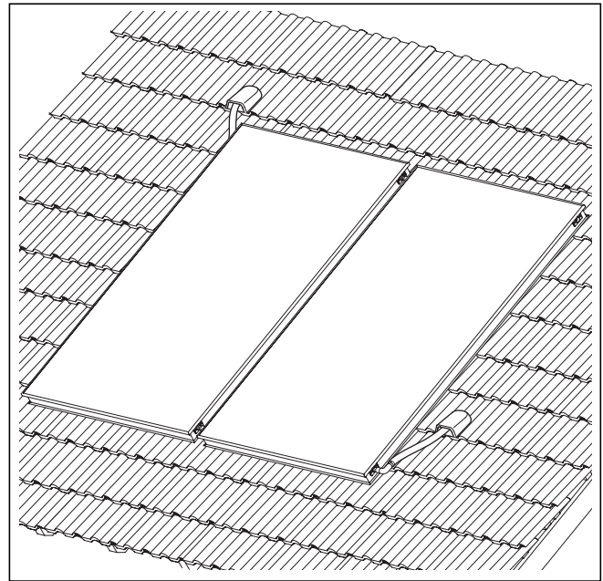
2.5 ábra Kétdarabos auroTHERM classic VFK 135 VD kollektor-mező (nem kapható minden országban) tetőre szerelve
