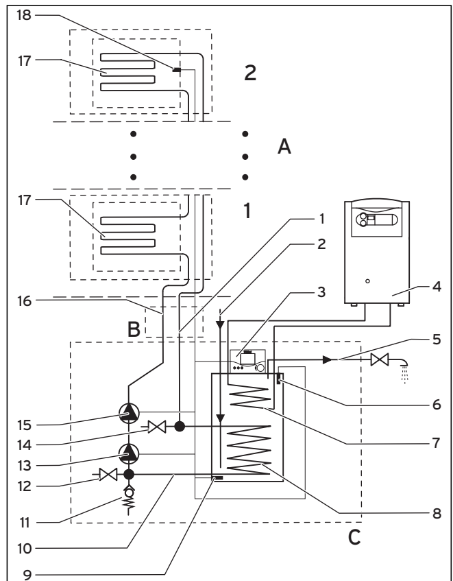
2.3 ábra VIH SN 250/3 iP tárolóval rendelkező auroSTEP plus rendszer fő komponensei (elvi vázlat csatlakozótartozékok nélkül)
