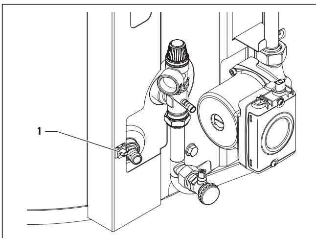
4.2 ábra A használati melegvítartó üritőszelepe
