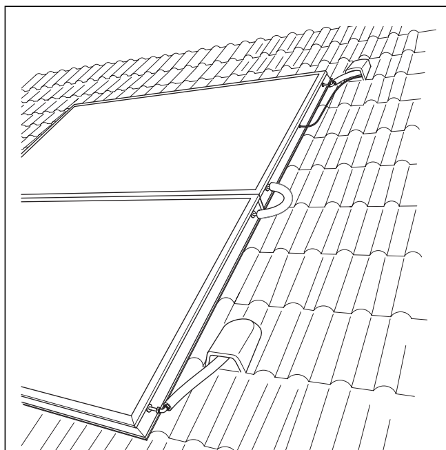
2.4 ábra Kétdarabos auroTHERM classic VFK 135 D kollektormező tetőre szerelve
