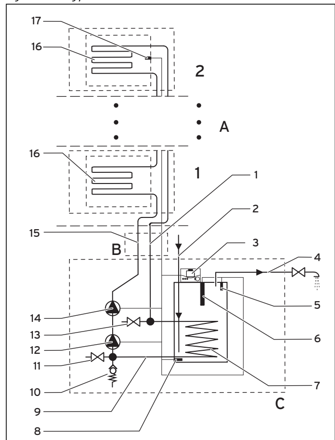
2.3 ábra Az auroSTEP plus készülékből és VEH SN 150/3 i tárolóából álló rendszer fő komponensek (elvi vázlat a csatlakozási tartozékok nélkül)
