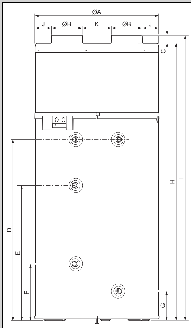
Készülékmeretek és csatlakozási méretek 200 és 270 l esetén
