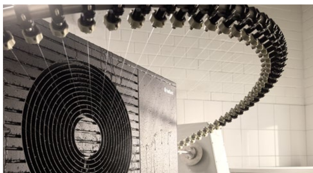
Vízugaras teszt az extrém esőzések elleni védelemhez
